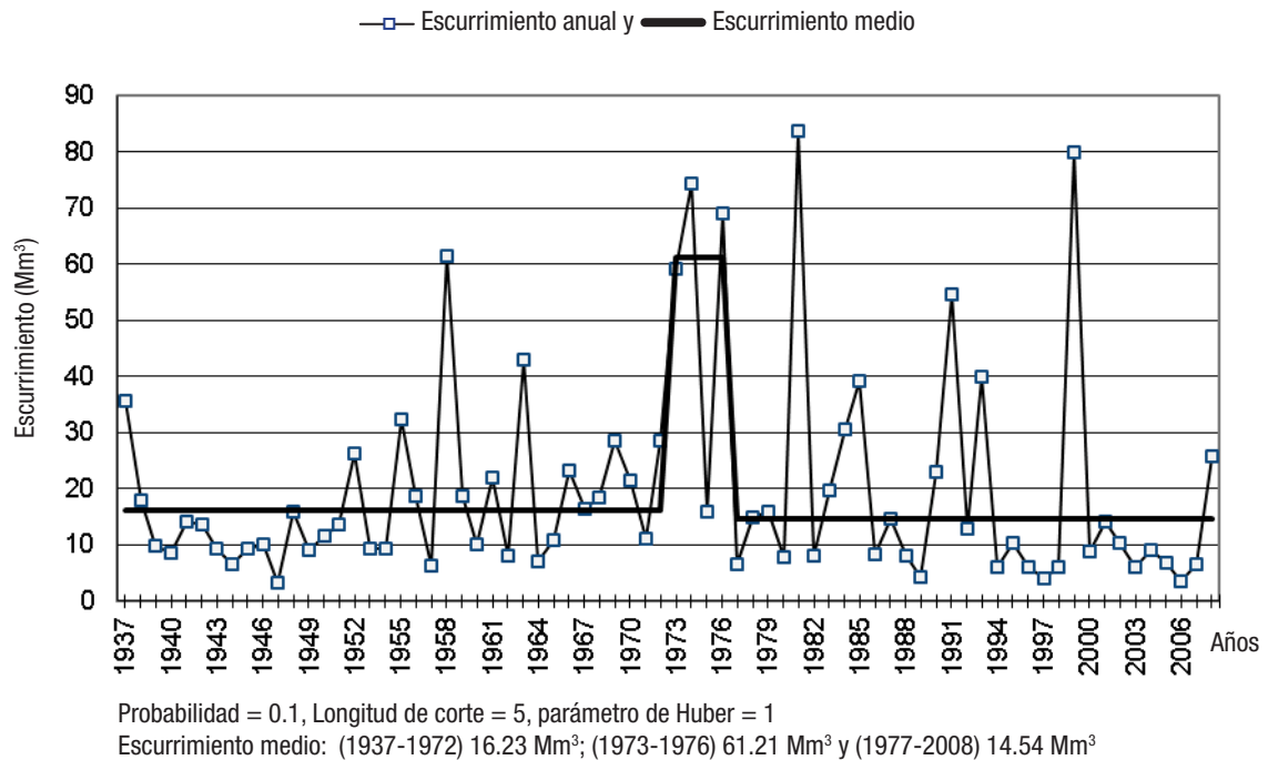
Figura 5. Cambios en el régimen de los escurrimientos medios de julio (1937-2008) de la cuenca Metztlitlán, en Hidalgo, México (longitud de corte: 5 años).
