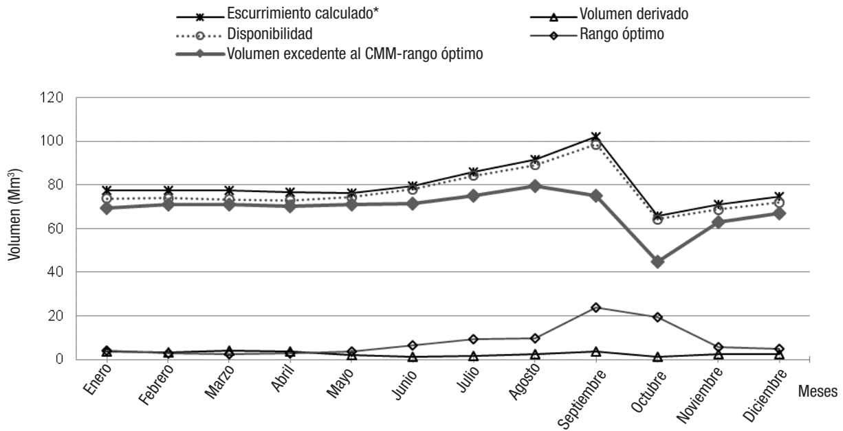
Figura 7. Volúmenes de desfogue excedentes al caudal ambiental de rango óptimo del lago de Metztlán, en Hidalgo, México. *Con probabilidad empírica de 80%.
