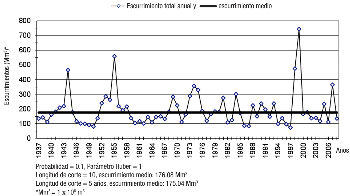
Figura 2. Régimen de escurrimientos totales anuales (1937-2008) de la cuenca Metztlitlán, en Hidalgo, México.
