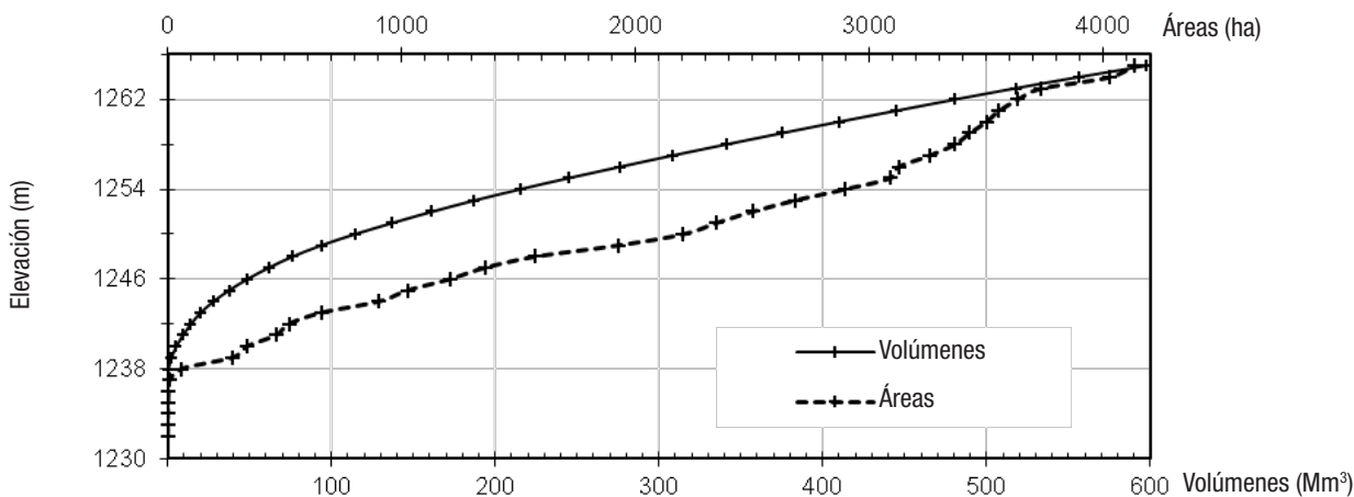
Figura 6. Curvas de elevaciones-áreas-capacidades para el lago de Metztlitlán, en Hidalgo, México.
